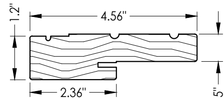
1A WOOD JAMB FrameSaver (Endura)
