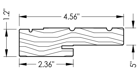
1 WOOD JAMB
